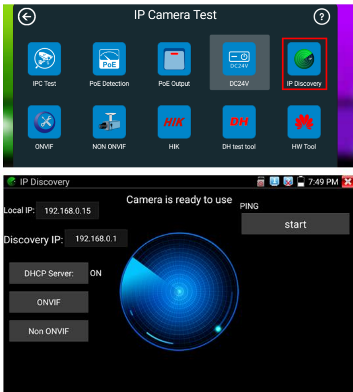
Рис.14 Приложение IP-Discovery
